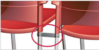
Pinça d'unió en Polipropilè de 5 mm de gruix
